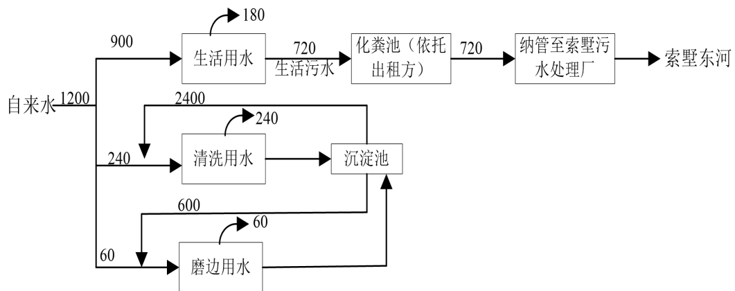
图 2-2 项目全厂水平衡图（单位：t/a）
