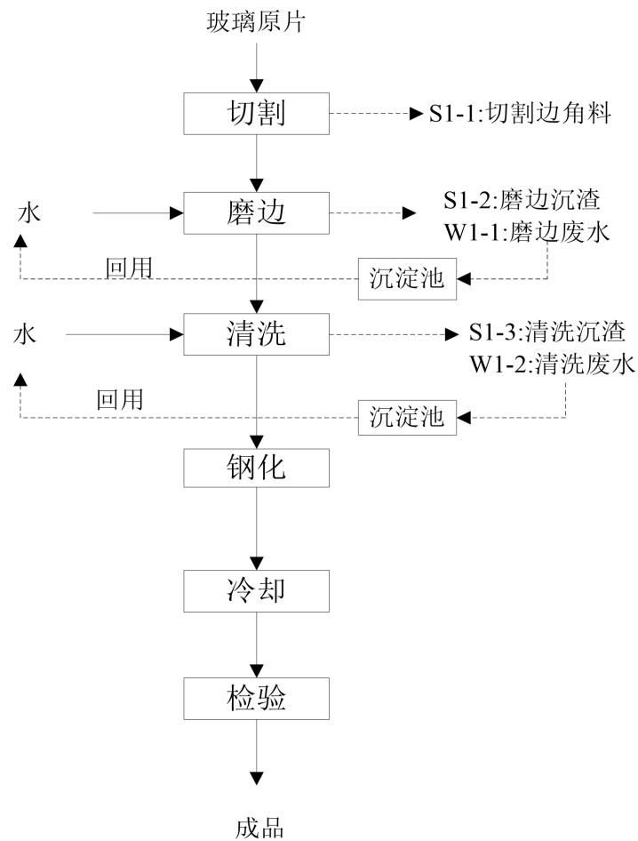
图 2-3 钢化玻璃工艺流程及产污环节图
