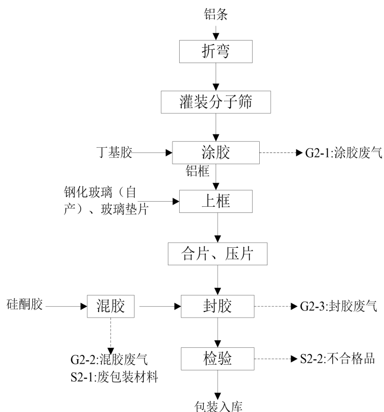
图 2-4 中空玻璃工艺流程及产污环节图
