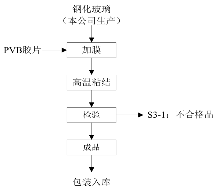
图 2-5 夹胶玻璃工艺流程及产污环节图
