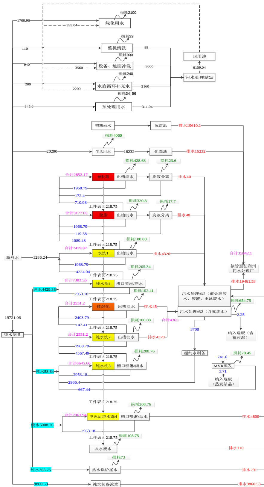
图 4-4 项目全厂水平衡图 (m³/a)
