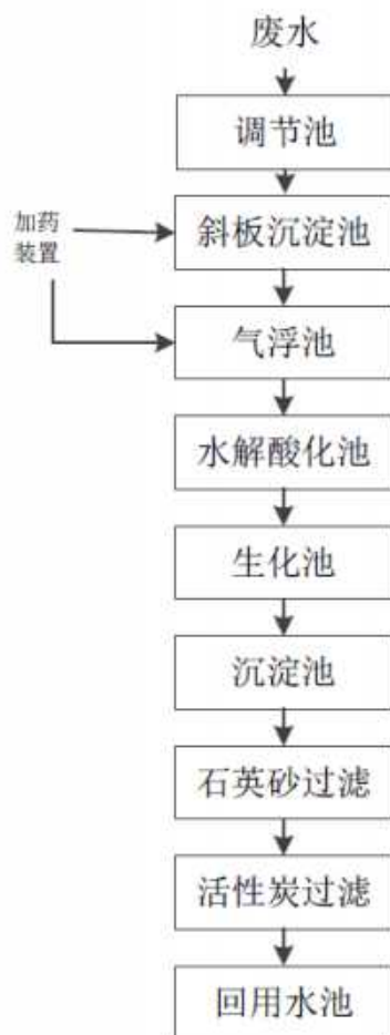
图 2-15 厂内污水处理站工艺流程图
