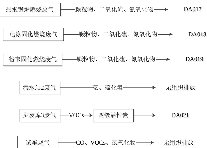
图 4-2 废气处理措施示意图
