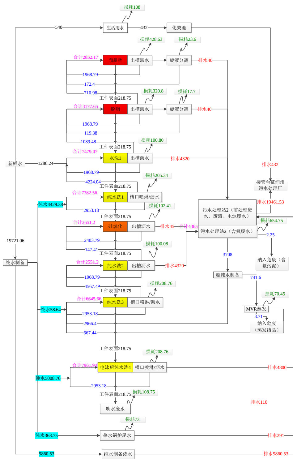
图 4-3 项目水平衡图 ( \text{m}^3/\text{a} )
