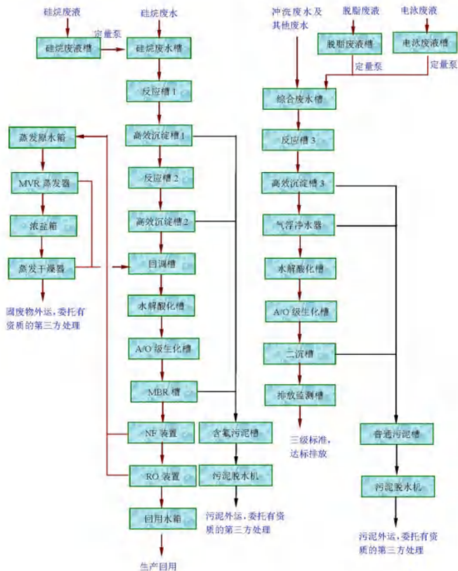
图 4-4 污水处理站 2#工艺流程图
