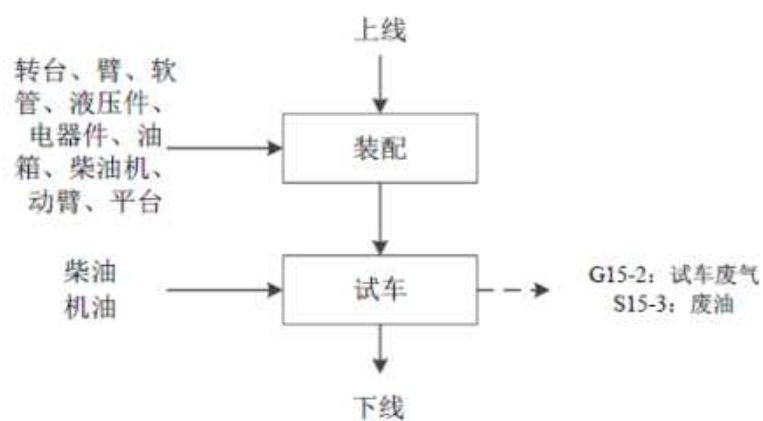
图 2-9 直臂式（柴油）作业平台装配工艺流程
