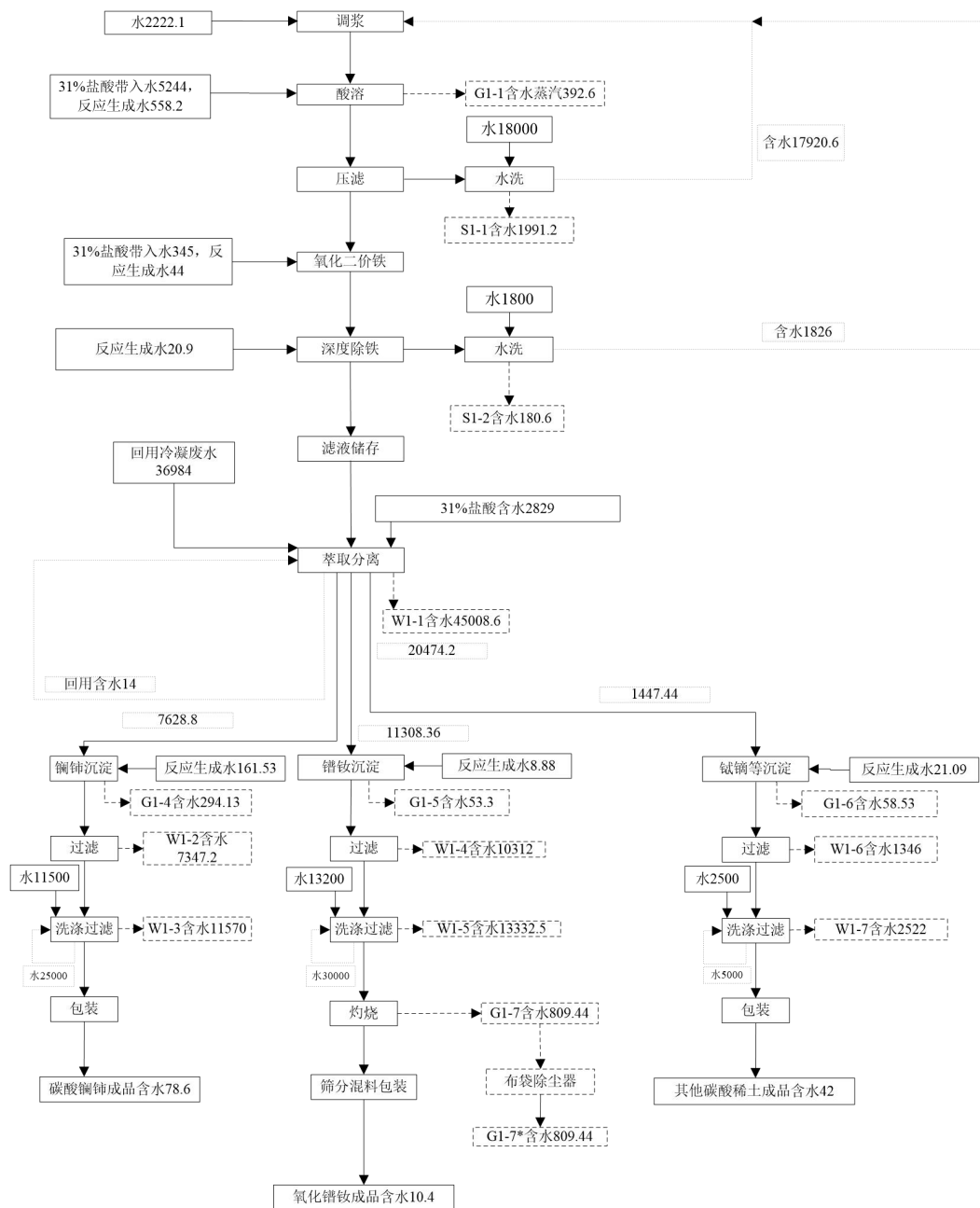
图 2.4-3 钕铁硼废料回收工艺水平衡图 (t/a)
