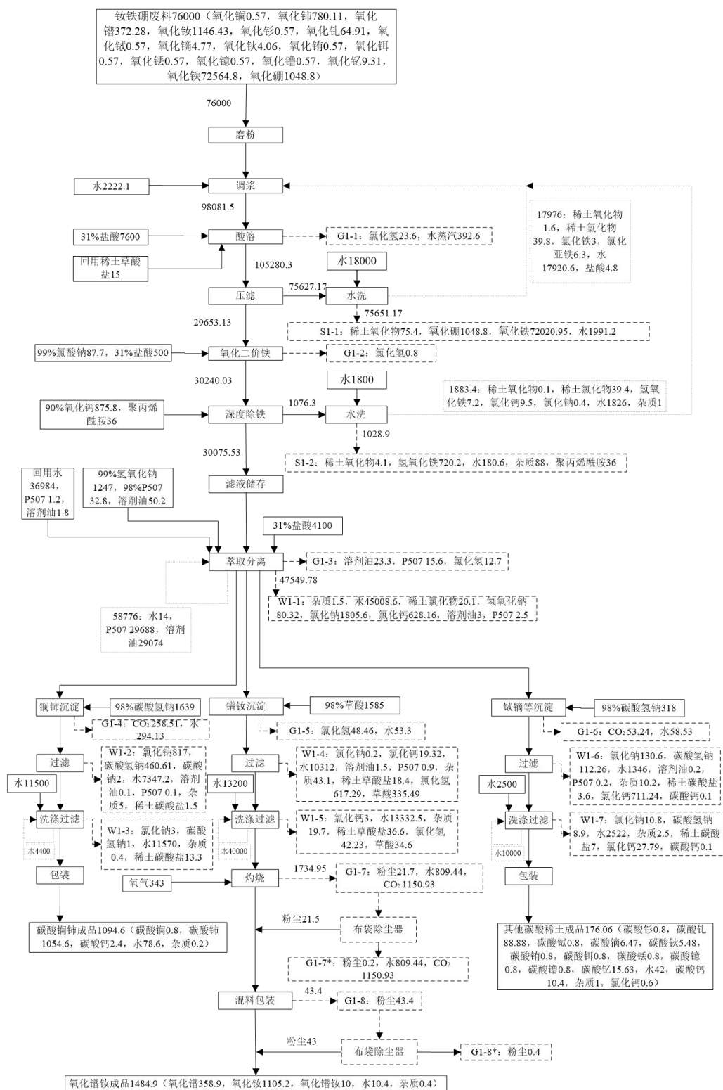
图 2.4-2 钕铁硼废料回收生产物料平衡图 (t/a)
