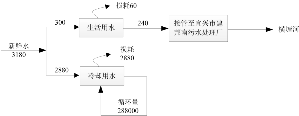
图 2.1-1 项目水平衡图（单位：m 3 /a）
