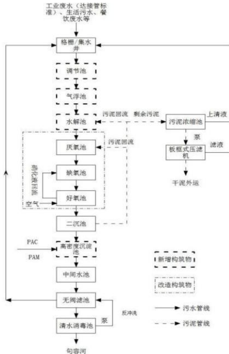
图 4-1 湖熟集镇污水处理厂工艺流程图
