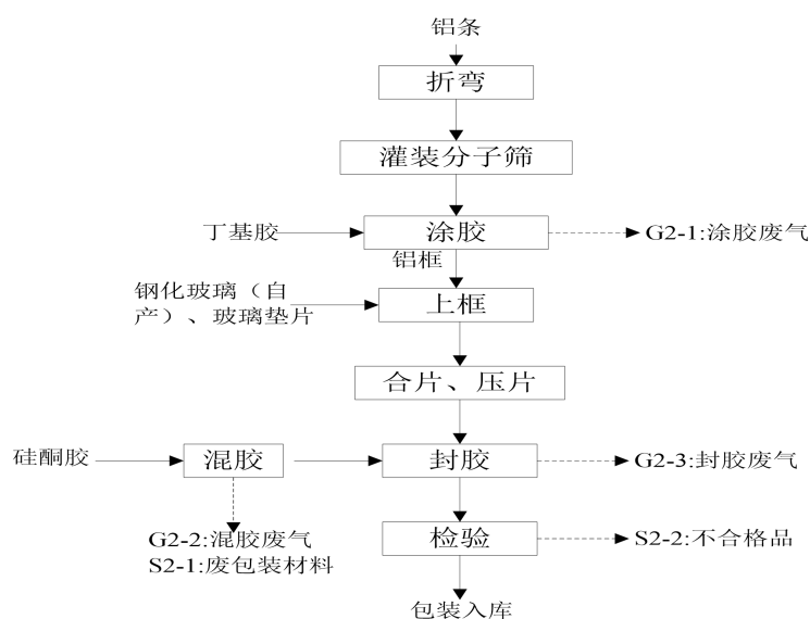
图 2-3 中空玻璃工艺流程及产污环节图
