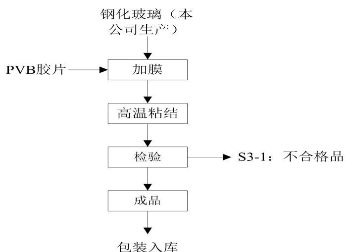
图 2-4 夹胶玻璃工艺流程及产污环节图 夹胶玻璃工艺流程简述：
