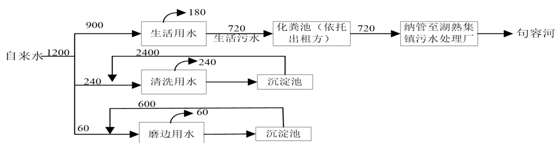
图 2-1 项目全厂水平衡图（单位：t/a）
