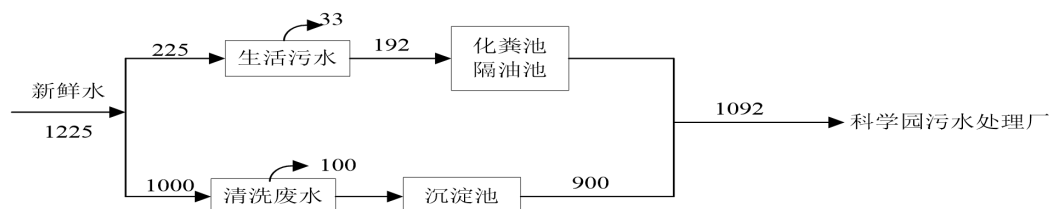
图 2-5 现有项目给排水平衡图（单位：t/a）
