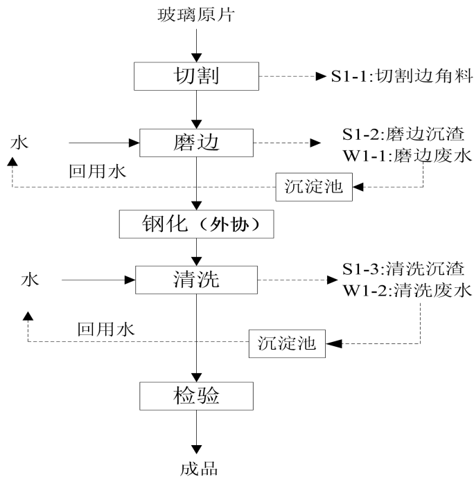
图 2-2 钢化玻璃工艺流程及产污环节图
